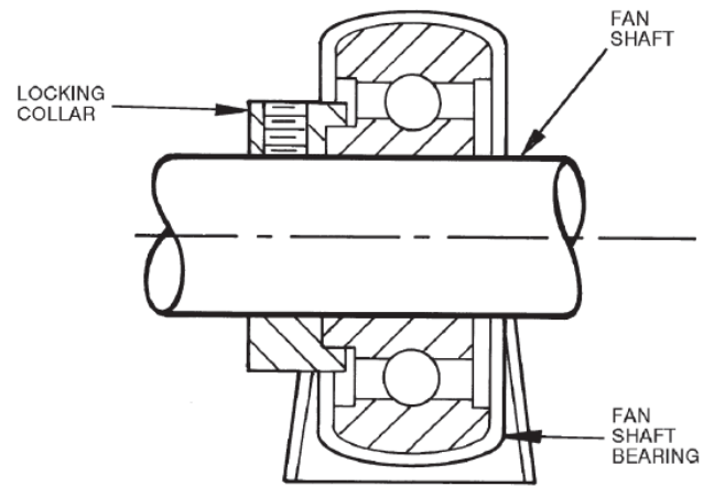
Fan Shaft Bearing
